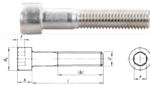
Zylinderschrauben mit Innensechskant nach DIN 912 in A2
