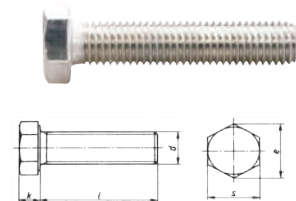
Sechskantschrauben mit Gewinde nach DIN 933 in A2
