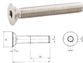
Senkschrauben mit Innensechskant nach DIN 7991 in A2
