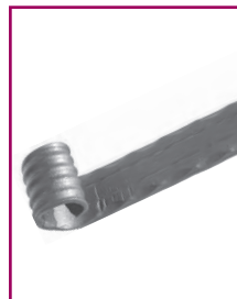
Handlauf-Ende 140 x 60 mm Best.-Nr. 7027 Aus 40 x 8 mm, 0,47 kg
